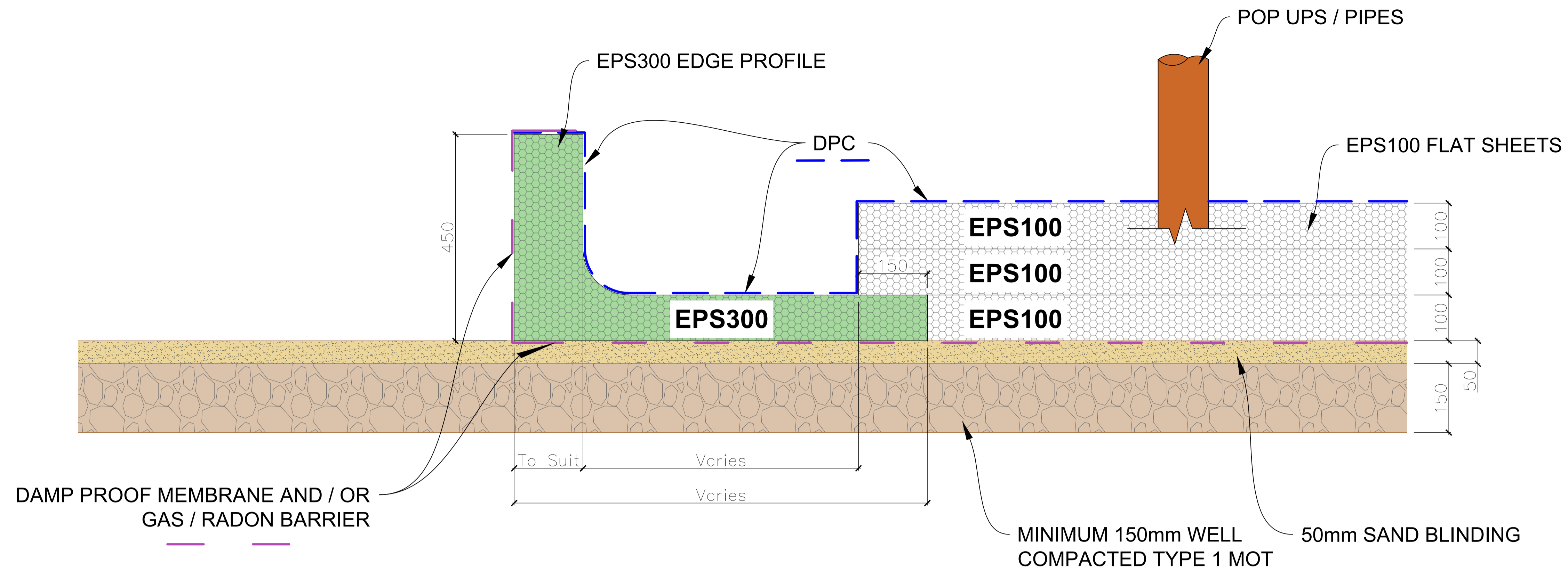
TYPICAL ICF WALL EDGE SECTION - BEFORE CONCRETE POUR
